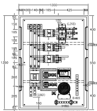
佈置圖
