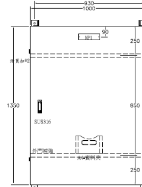
正視圖
