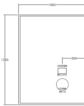
中門開孔圖
