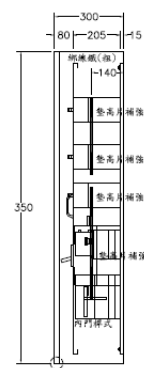
右側視圖
