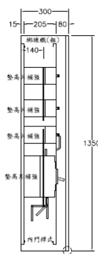
左側視圖
